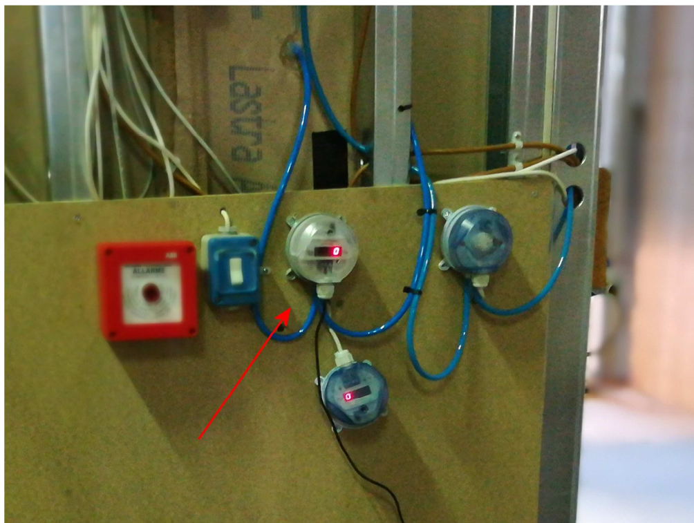
Fotografia del trasmettitore di pressione differenziale dell'Istituto Giordano
