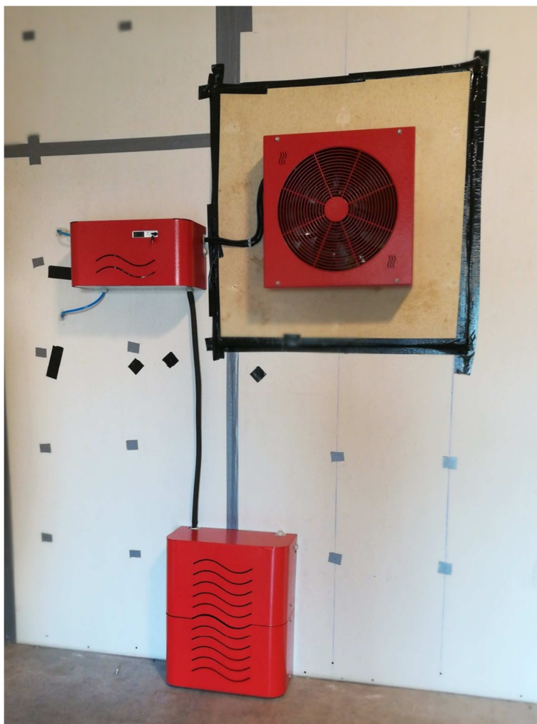
Fotografia del sistema di pressurizzazione
