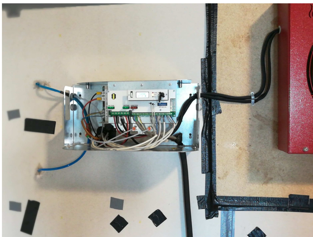
Fotografia dell'interno della scatola superiore dell'unità di comando dove è presente la scheda di gestione del sistema
