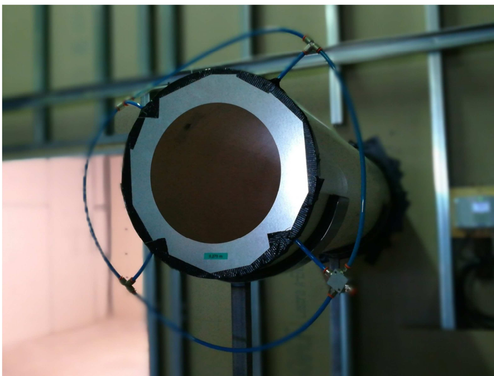
Fotografia della flangia di riduzione posta all'estremità del canale d'aspirazione
